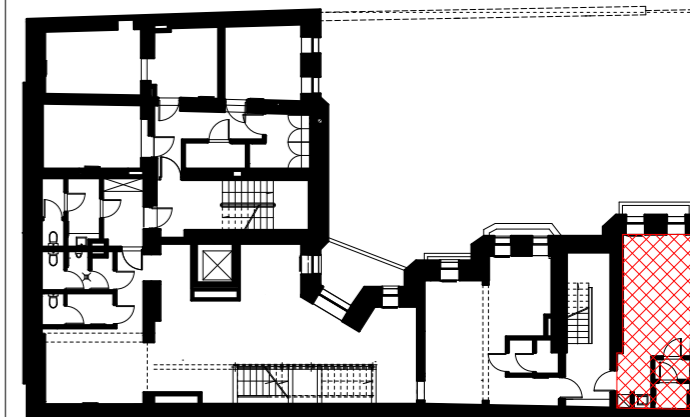
SCHEMAT PIWNICY
