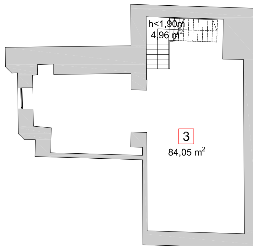
RZUT PIWNICY
