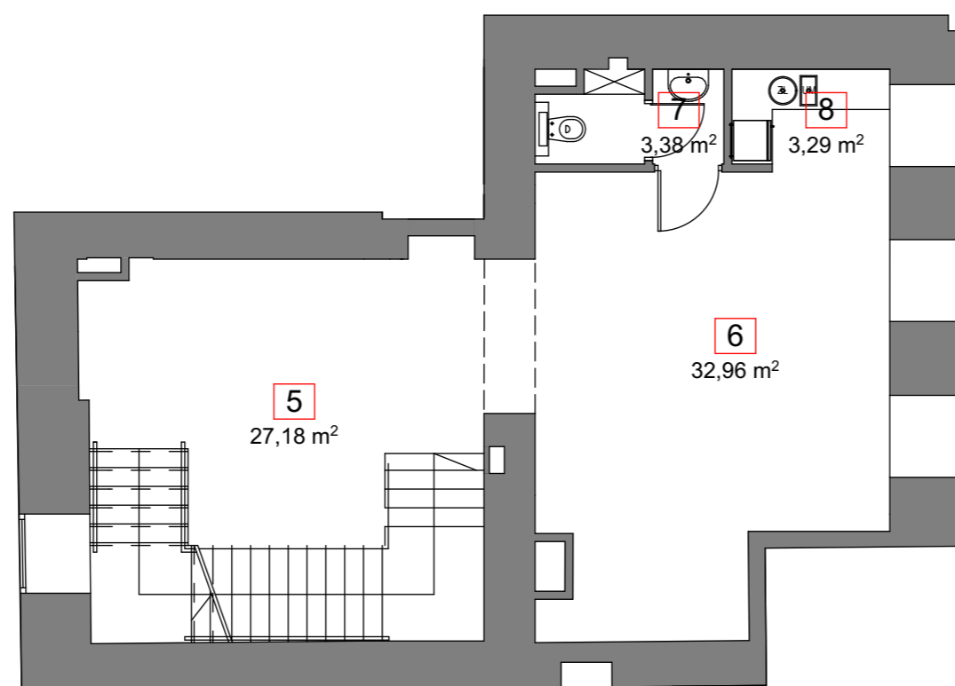
RZUT PIWNIC
